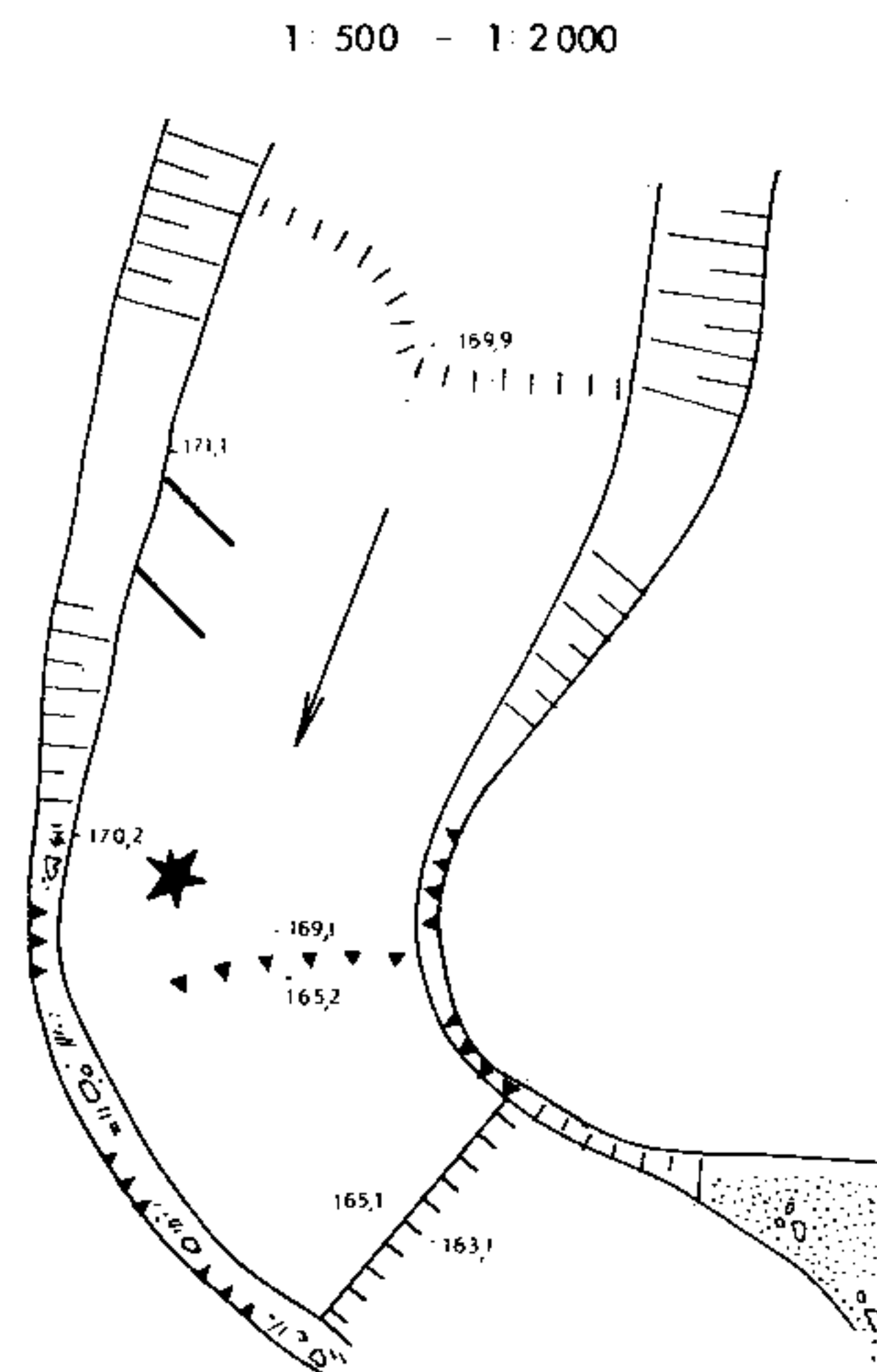
81. Primjer crtanja prirodnog vodotoka sa stalnom vodom
